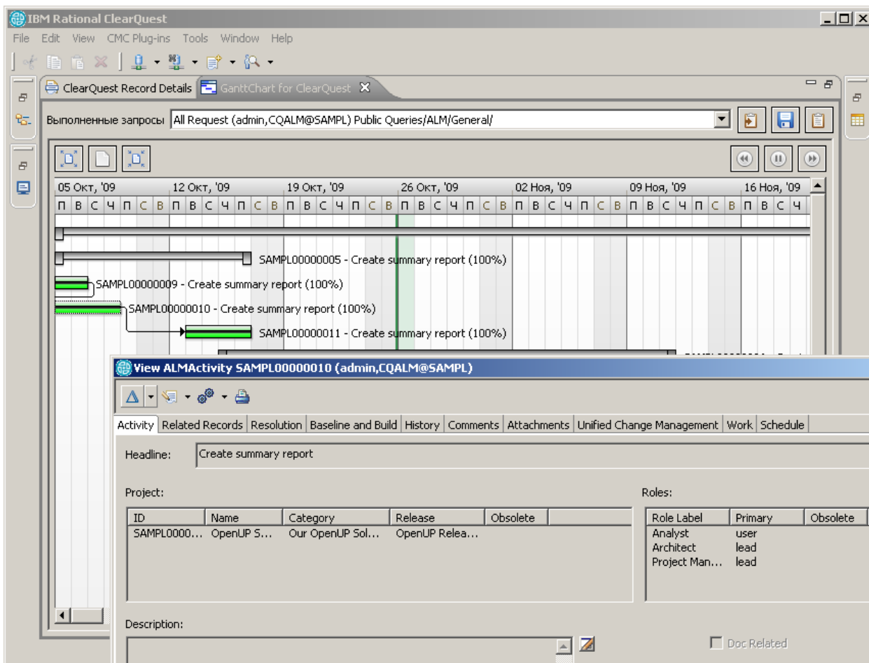
Рисунок 13. Открытая форма из диаграммы Ганта
