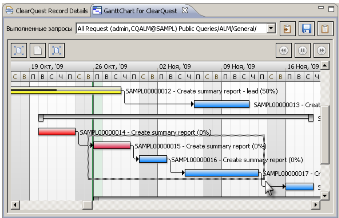
Рисунок 14. Выделение группы задач
