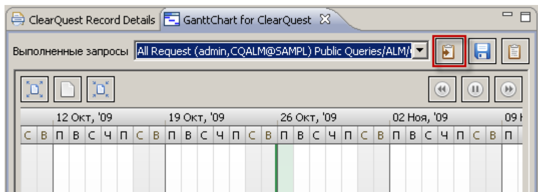
Рисунок 11. Выполнение запроса
